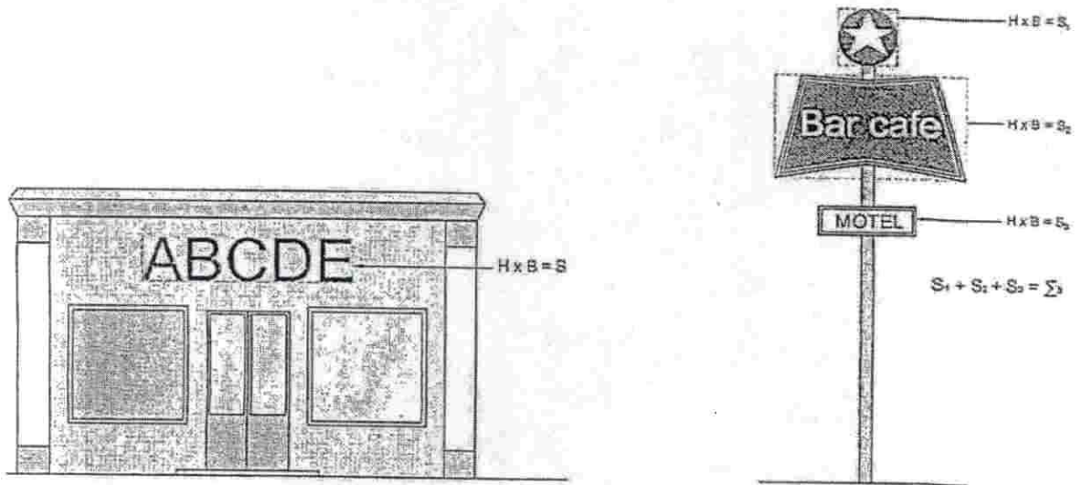
Hình A.1 - Phương tiện quảng cáo dạng chữ gắn trực tiếp lên mặt ngoài công trình
